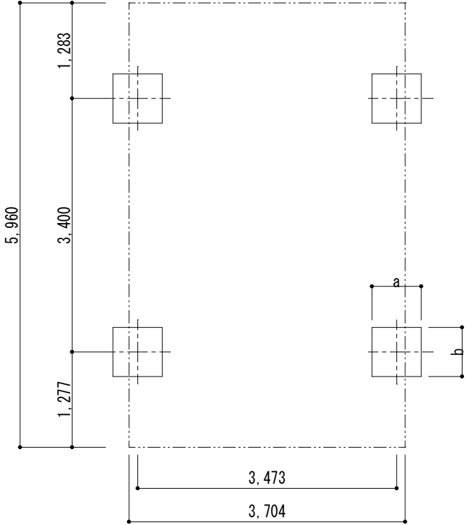
■ 基礎配置図
